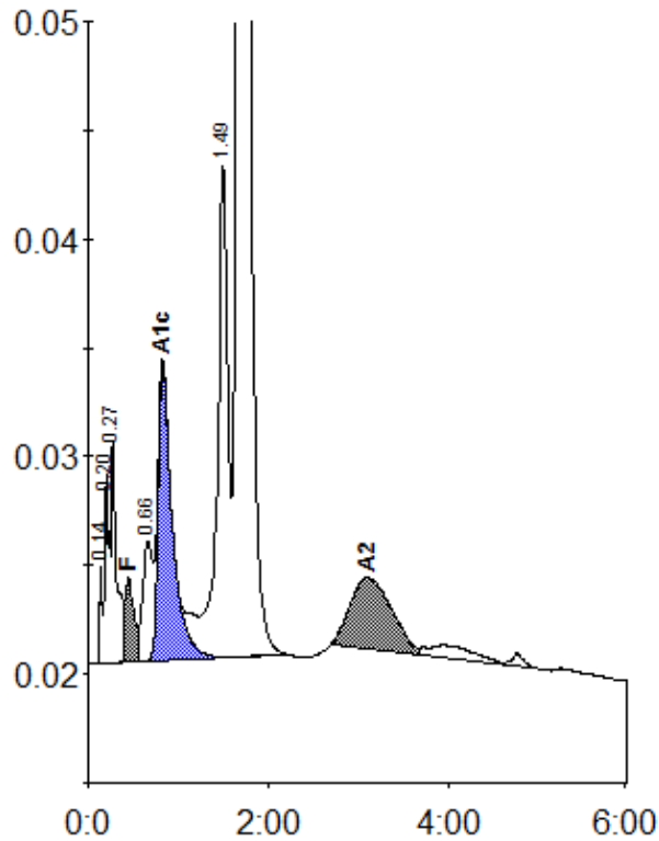
Peak table - ID: 06030026
