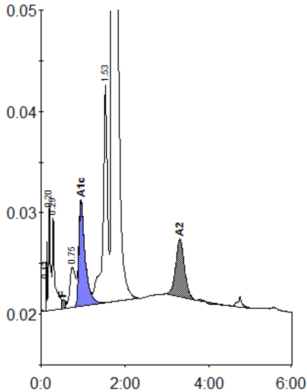
Peak table - ID: WCD13869
